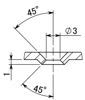
断面図 A-A 詳細図B S=2/1
