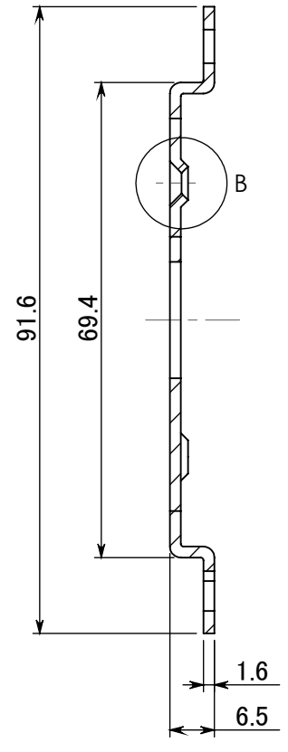
断面図A-A
