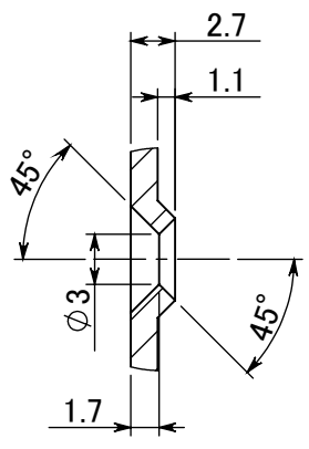
詳細図B S=2/1
